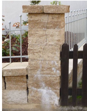
Bild 3: Torsäule mit Rissebildung und Kalkausblühungen - verursacht durch Arbeits- und Materialfehler.
